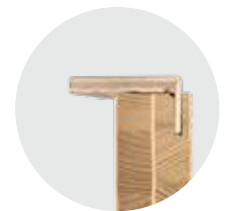
Huisserie en contre-plaqué, couvre-joints en multiplis
